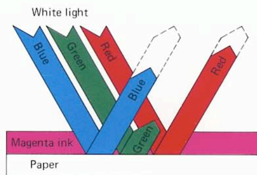
(d) Actual absorption and reflection qualities of magenta ink.
